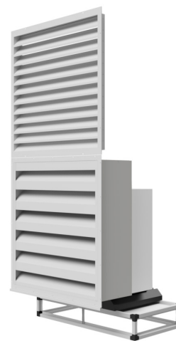
Tekening 3: Warmtepomp opstelling met geluidswerend buitenluchtrooster WGA
