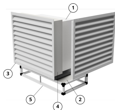
Tekening 2: Warmtepomp opstelling - buitenluchtroosters naast elkaar
