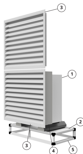
Tekening 1: Warmtepomp opstelling - buitenluchtroosters boven elkaar
